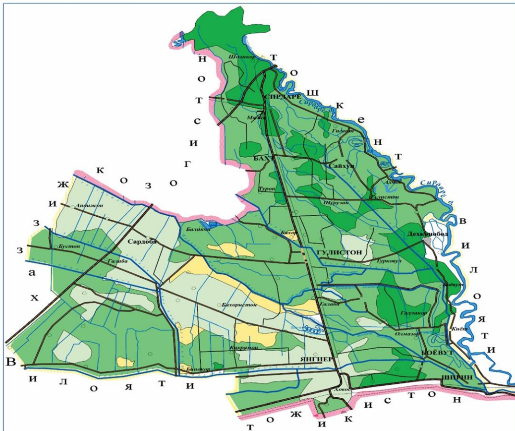
4-расм. СИРДАРЁ ВИЛОЯТИ АГРОЭКОЛОГИК ХАВФЛИЛИК КАРТАСИ
