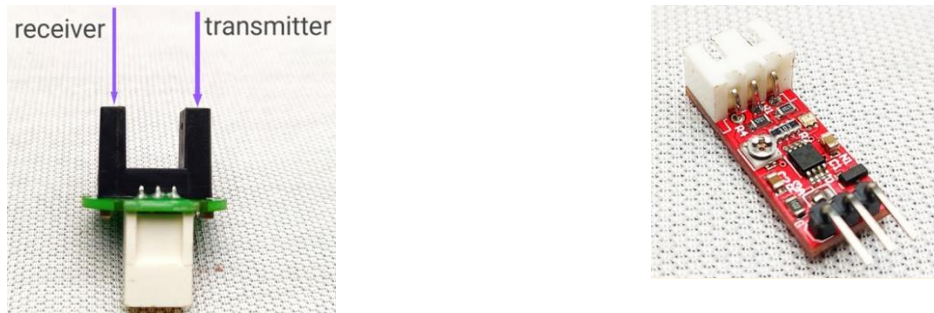
Рис. 1. Датчика мутности
