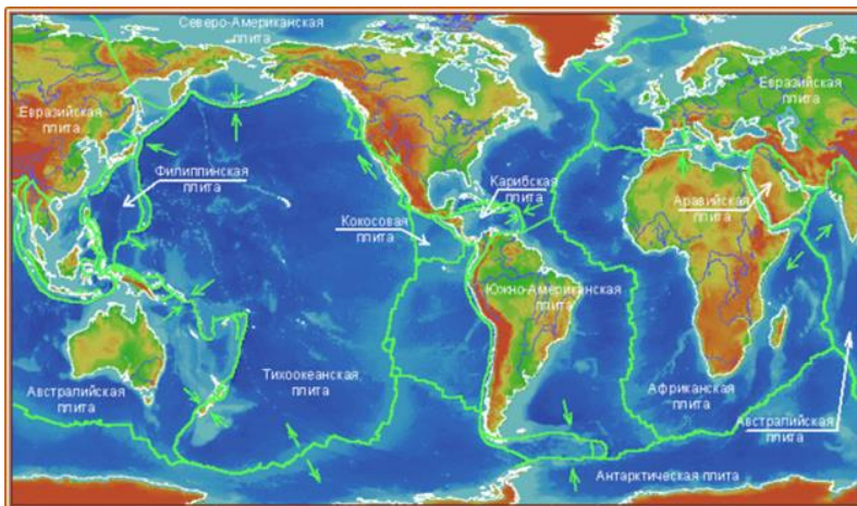
Ер шарининг сейсмик камари
